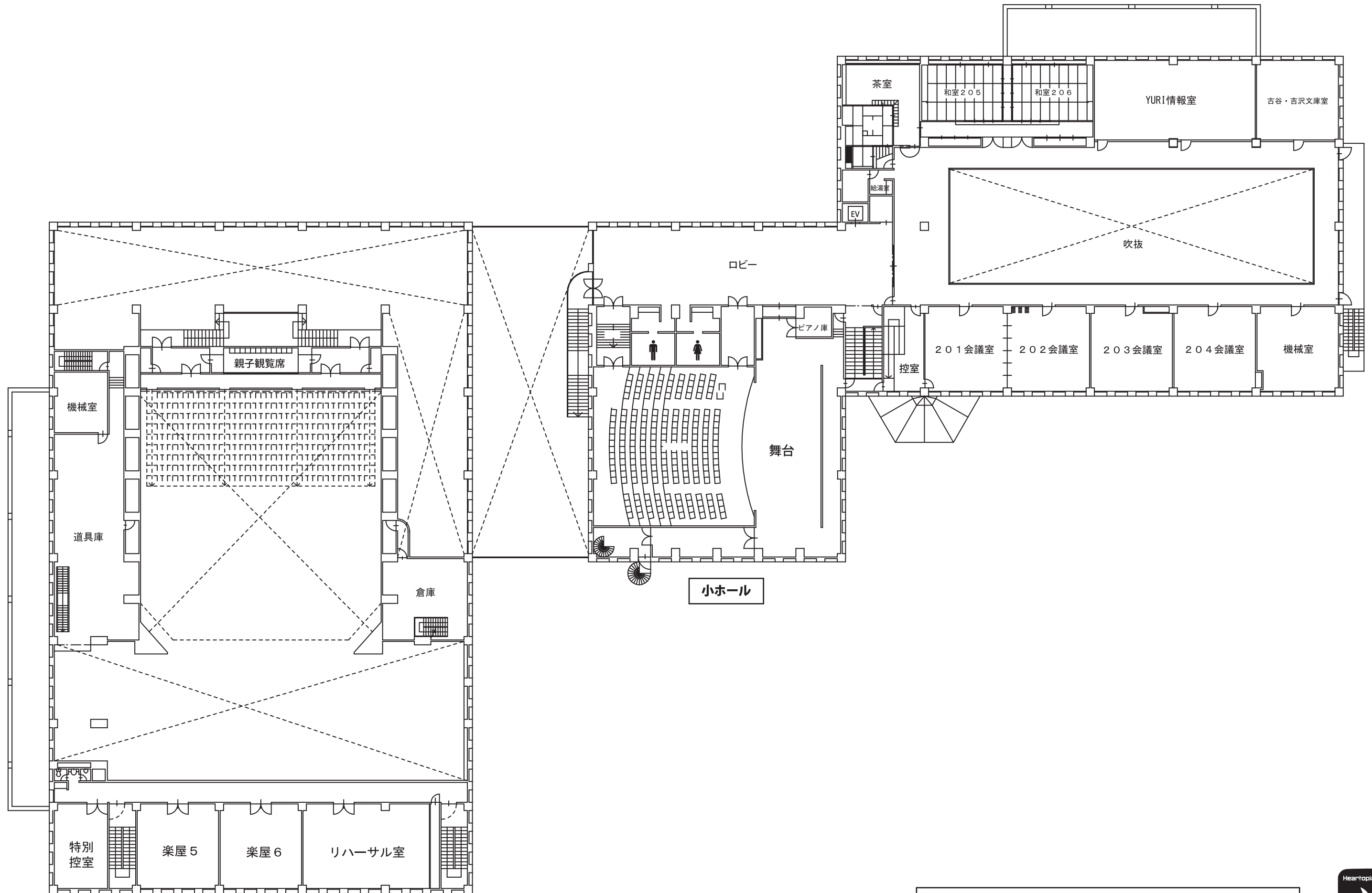
ハートピア春江 2F平面図
